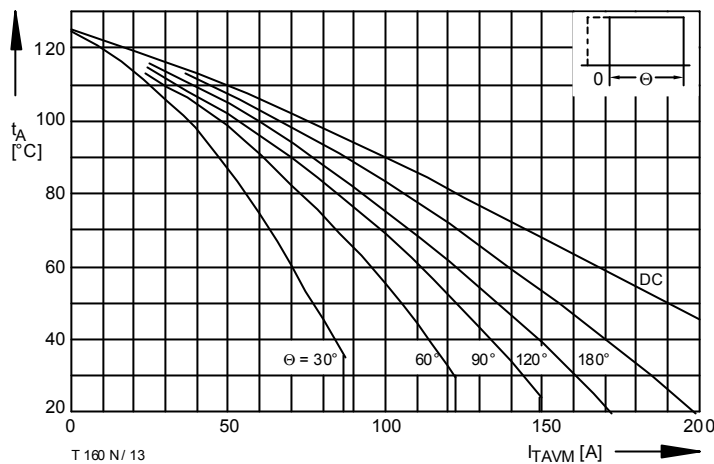
Bild / Fig. 13 Höchstzulässige Kühlmitteltemperatur / Max. allowable cooling medium temperature t_A = f(I_{TAVM}) Verstärkte Luftkühlung / Forced air-cooling, V_L = 50 l/s Kühlkörper / Heatsink: K0.55-M12-A, V_L = 50 l/s Parameter: Stromflußwinkel / Current conduction angle \theta
