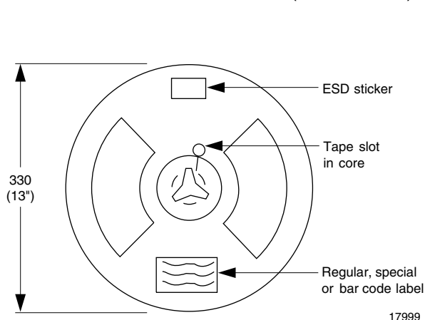
Fig. 6 - Reel Dimensions
