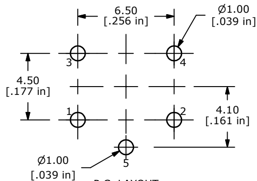
P.C. LAYOUT
