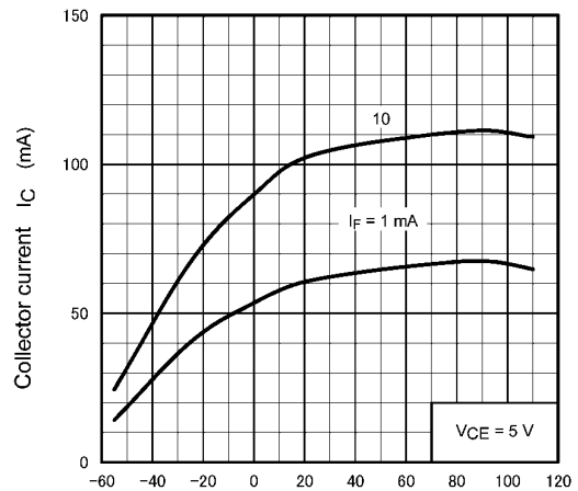
Fig. 11.12 I_C - T_a
