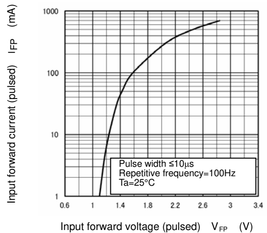
I_{FP} - V_{FP}
