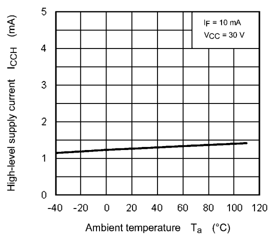
Fig. 13.2.6 I_{CCH} - T_a
