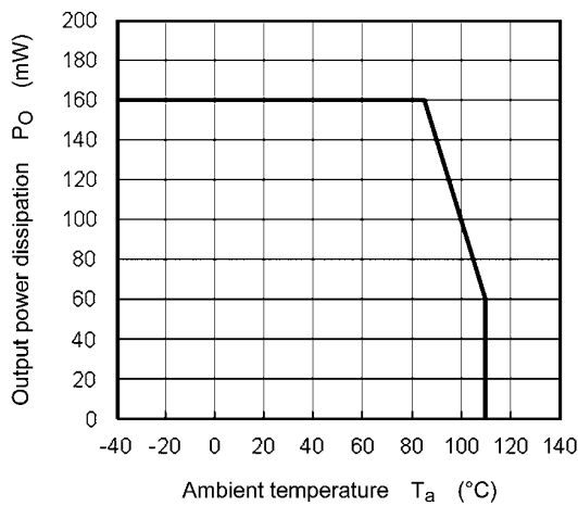
Fig. 13.2.3 P_O - T_a
