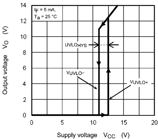
Fig. 13.2.11 V_o(V_{UVLO}) - V_{CC}
