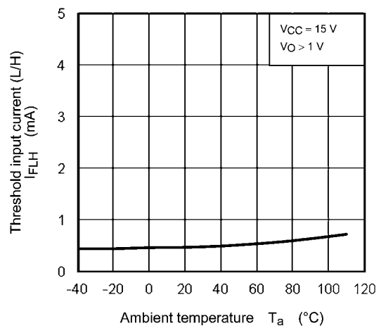
Fig. 13.2.4 I_{FLH} - T_a
