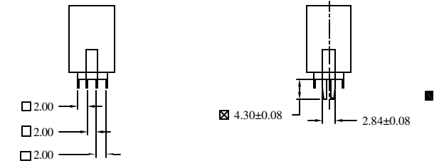
SECTION V-V
