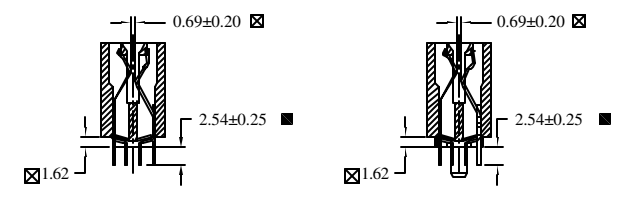
SECTION V-V
