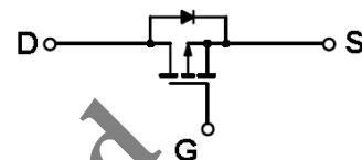
P-Channel MOSFET
