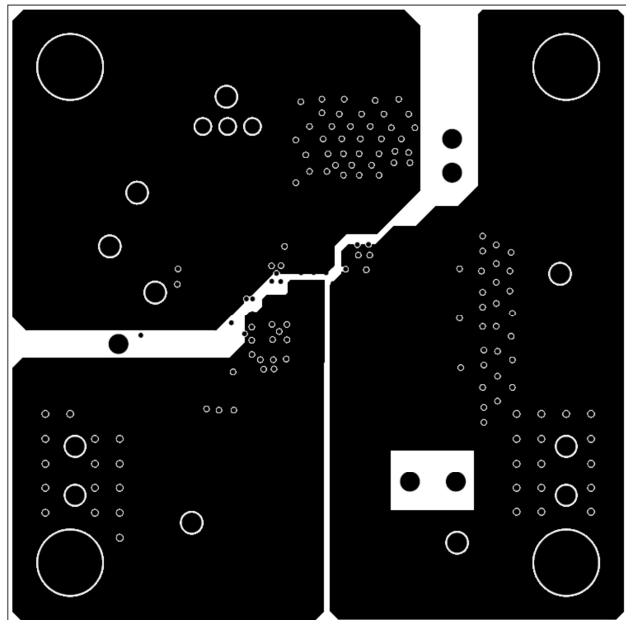
Fig. 10: Layer 5, VCC2
