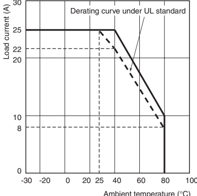
G3PB-225B-3-VD G3PB-225B-2-VD
