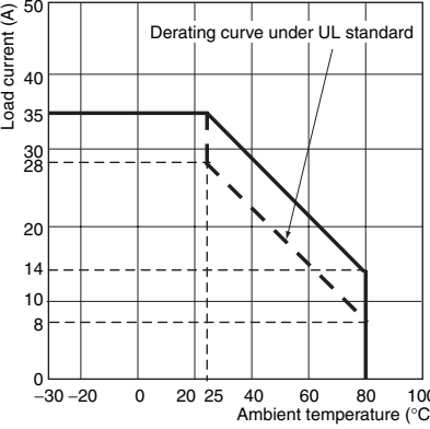
G3PB-235B-3-VD G3PB-235B-2-VD
