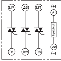
G3PB-245B-3-VD
