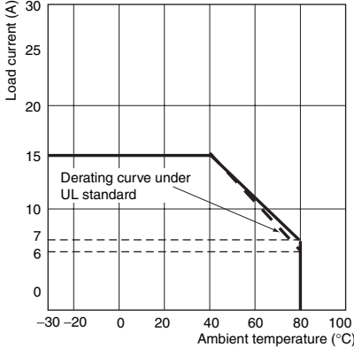
G3PB-215B-3-VD G3PB-215B-2-VD
