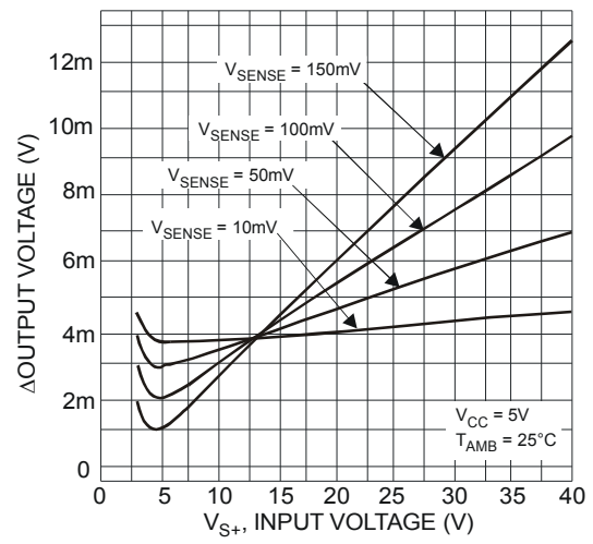
Fig. 10 Output Voltage
