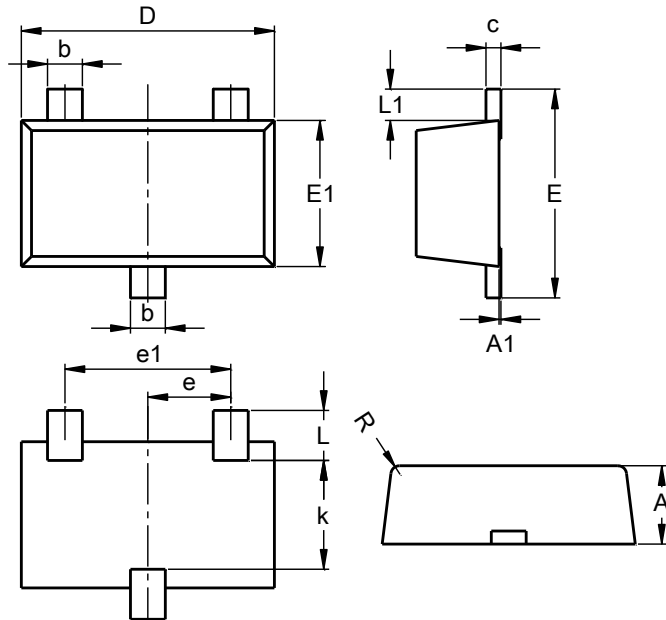
SOT23F
